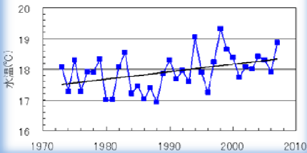
大阪湾の表層水温の年平均推移
