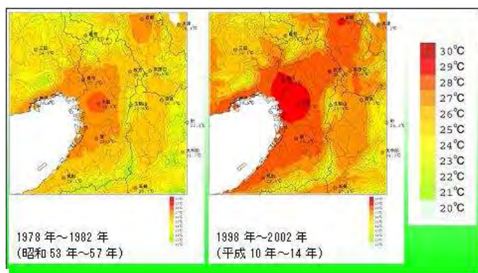
近畿地方の8月の平均気温分布(大阪管区気象台)
